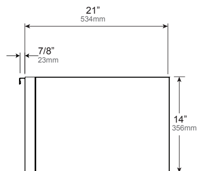
SLOW CLOSE ADD 7/8\" FERMETURE LENTE ADD 23MM SLOW CERRAR AGREGAR 23MM
