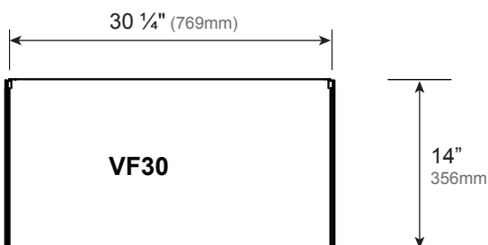
CROSS - SECTION WITH VFDRAWER COUPE TRANSVERSALE AVEC TIROIR VF SECCIÓN TRANSVERSAL CON CAJONERA VFD
