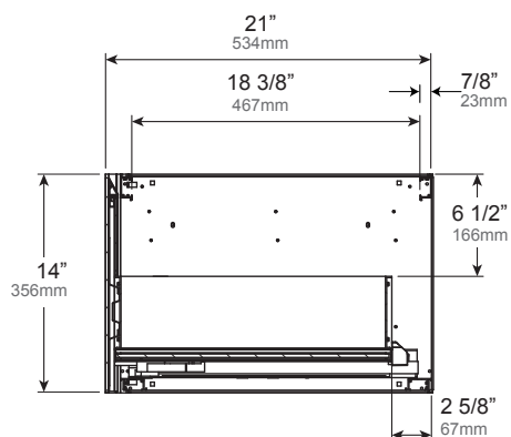
CROSS - SECTION WITHOUT VFDRAWER COUPE TRANSVERSALE VF SECCIÓN TRANSVERSAL SIN CAJONERA VFD
