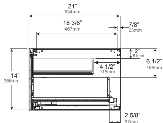
CROSS - SECTION WITH VFDRAWER COUPE TRANSVERSALE AVEC TIROIR VF SECCIÓN TRANSVERSAL CON CAJONERA VFD
