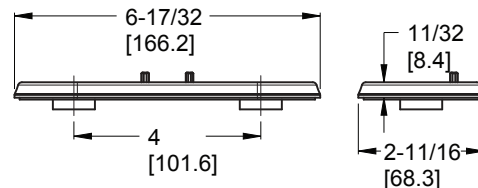
Optional Deckplate
