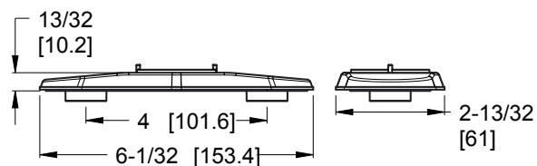
Optional Deckplate
