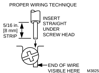
Fig. 4—Proper wiring technique.
