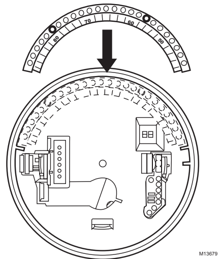
Fig. 3. Alineación del limitador de rango con el termostato.
