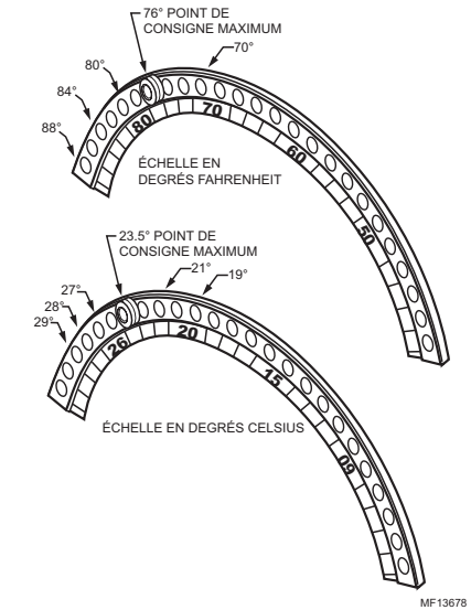
Fig. 5. Réglages de la butée de température maximale.
