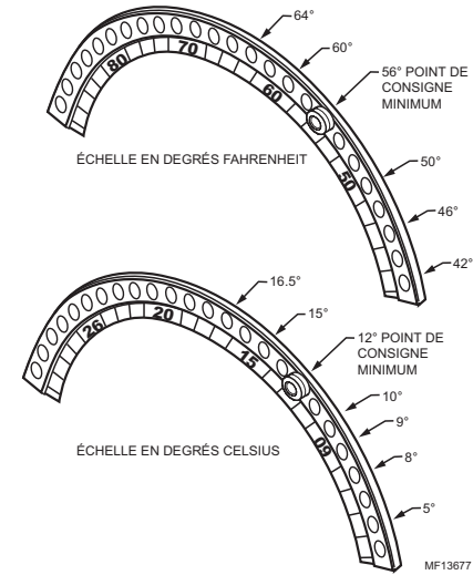
Fig. 4. Réglages de la butée de température minimale.
