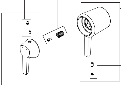
RP101943▲ Screw & Sleeve Tornillo y Manga Vis et Manchon
