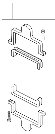
RP63688 Mounting Plates, Sleeves & Screws Chapas de instalación, Casquillos y Tornillos Plaques de montage, manchons et vis
