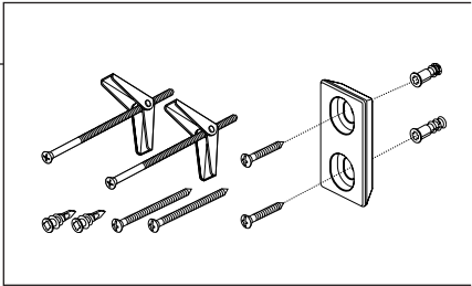
RP100215 Mounting Hardware Herraje de Instalación Pièces de montage
