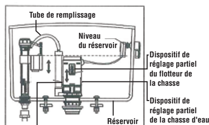
Dispositif de réglage complet de la chasse d'eau
