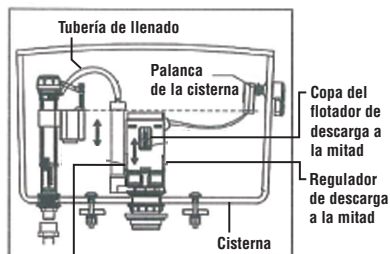
Regulador de vaciado completo
